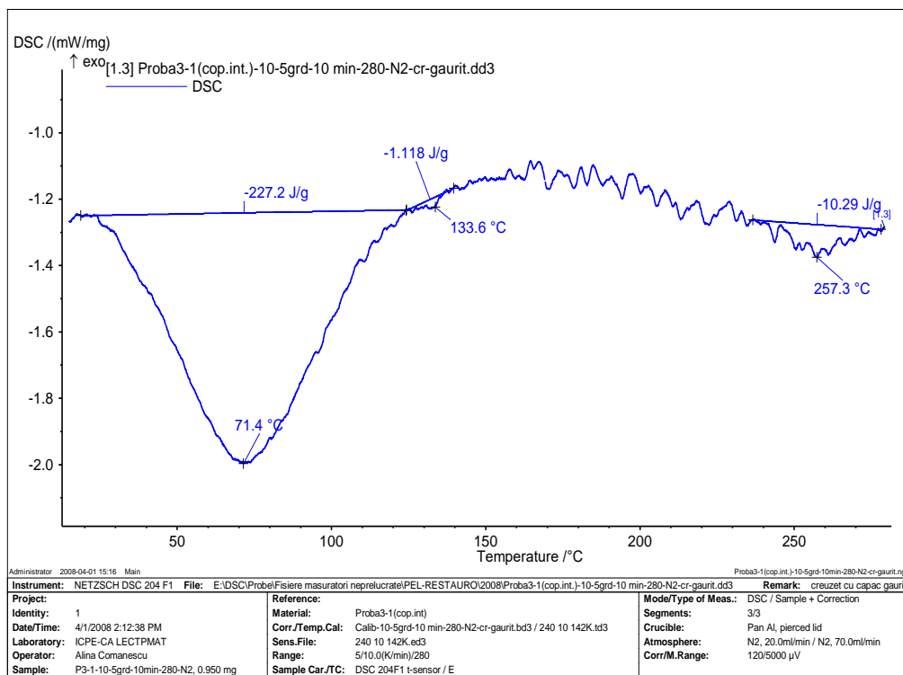
Fig. 1.7. Curba DSC pentru proba de piele P3-1
