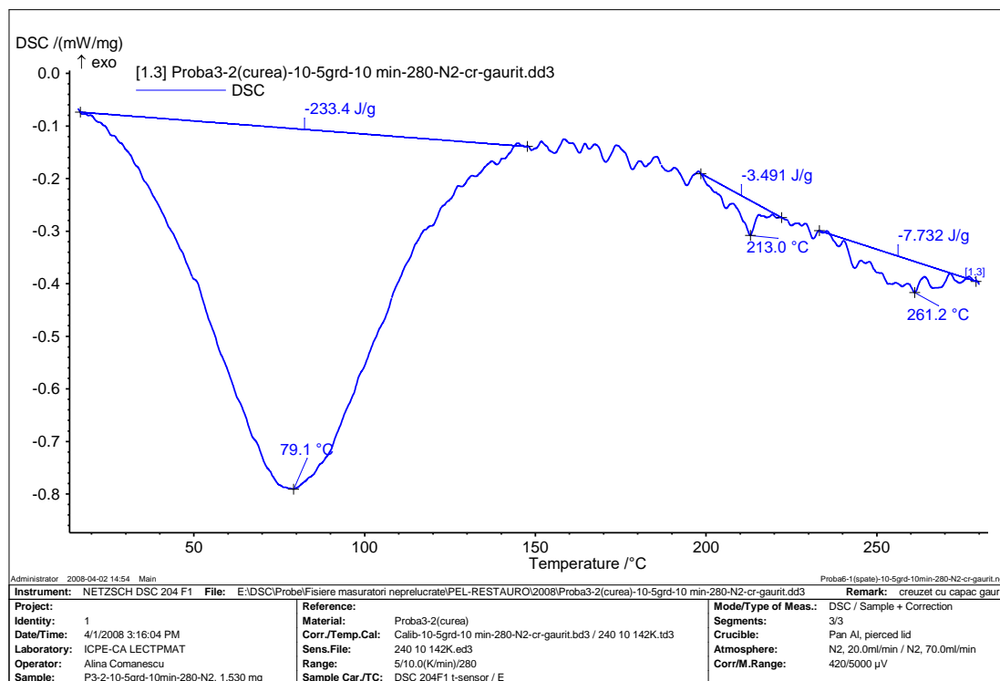
Fig. 1.8. Curba DSC pentru proba de piele P3-2
